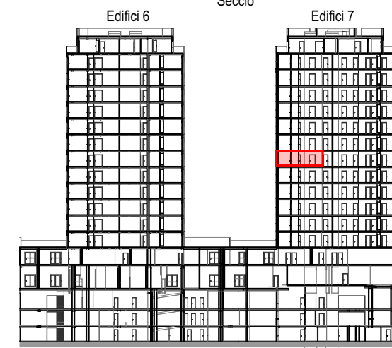
Secció
